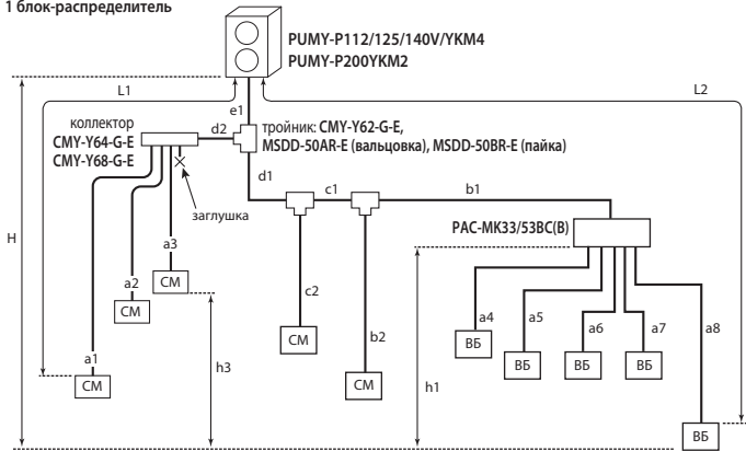
1 блок-распределитель
