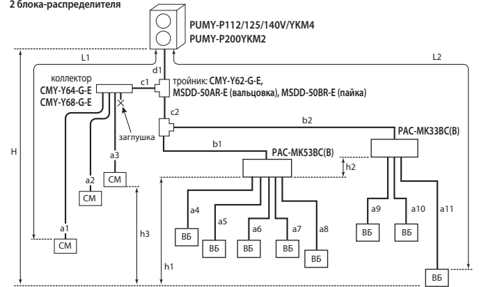
2 блока-распределителя
