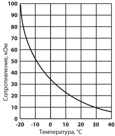
Термистор RT61: оттаивание Термистор RT65: наружная температура Термистор RT68: на теплообменнике
