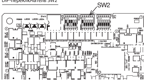
DIP-переключатель SW2
