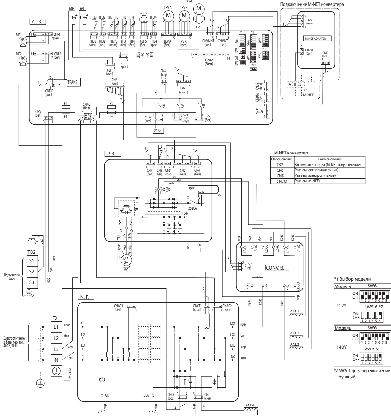
Подключение M-NET конвертера
