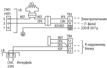
Рис. 1. Раздельное подключение электропитания к наружному и внутренним блокам.
