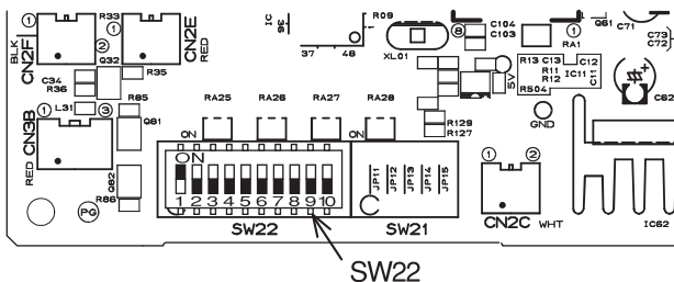
DIP-переключатель SW22
