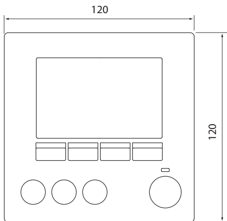
Вид спереди
