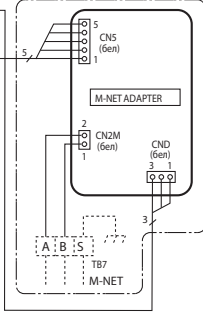
Подключение M-NET конвертера
