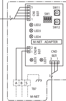
Конвертер для сети M-NET (Сити Мульти)
