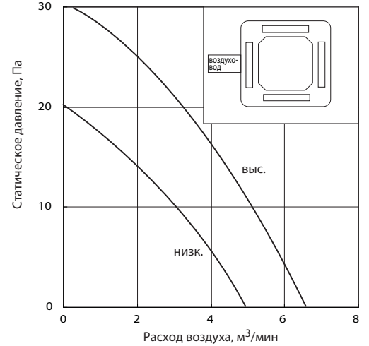
● 4 потока (заслонка - горизонтально). Прямоугольный воздуховод.
