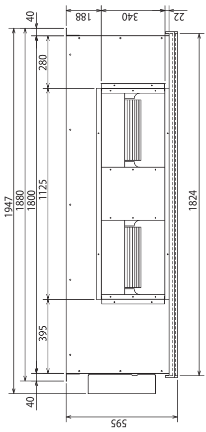
Вид спереди
