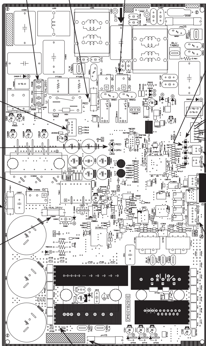
Термистор RT61: оттаивание Термистор RT65: наружная температура Термистор RT68: на теплообменнике
