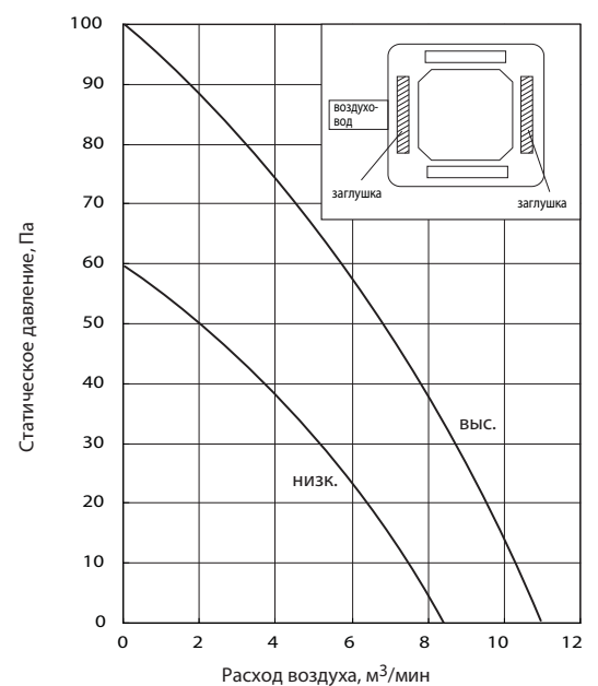
● 2 потока (заслонка - горизонтально). Прямоугольный воздуховод.
